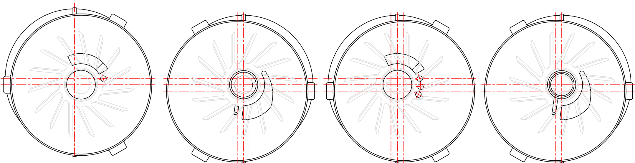
Közdarab első/front spacer 51 424 106
